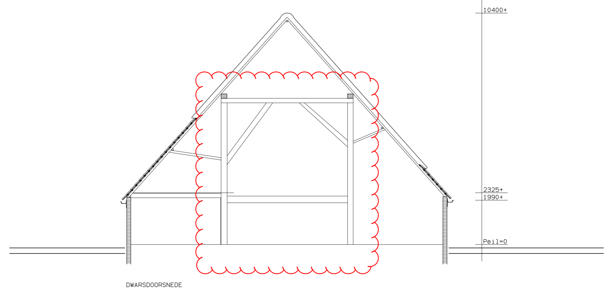
DWARSDOORSNEDE
