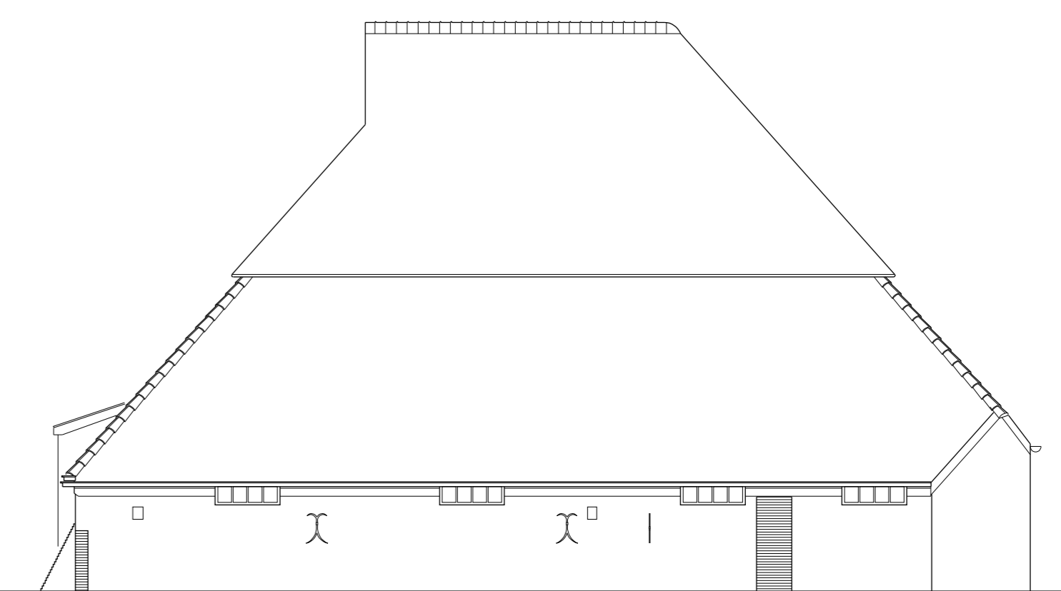
OOSTGEVEL
