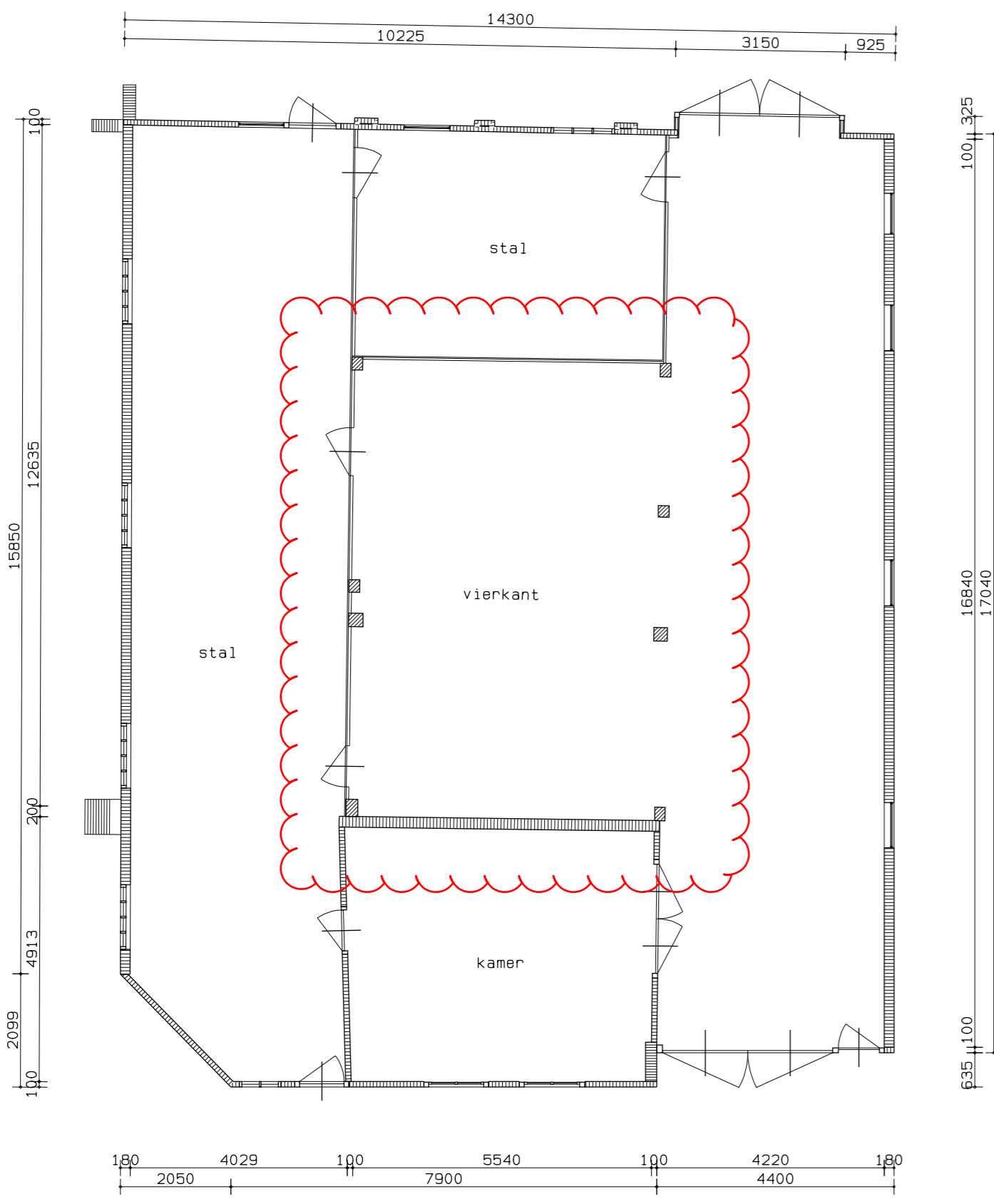
BEGANE GROND
